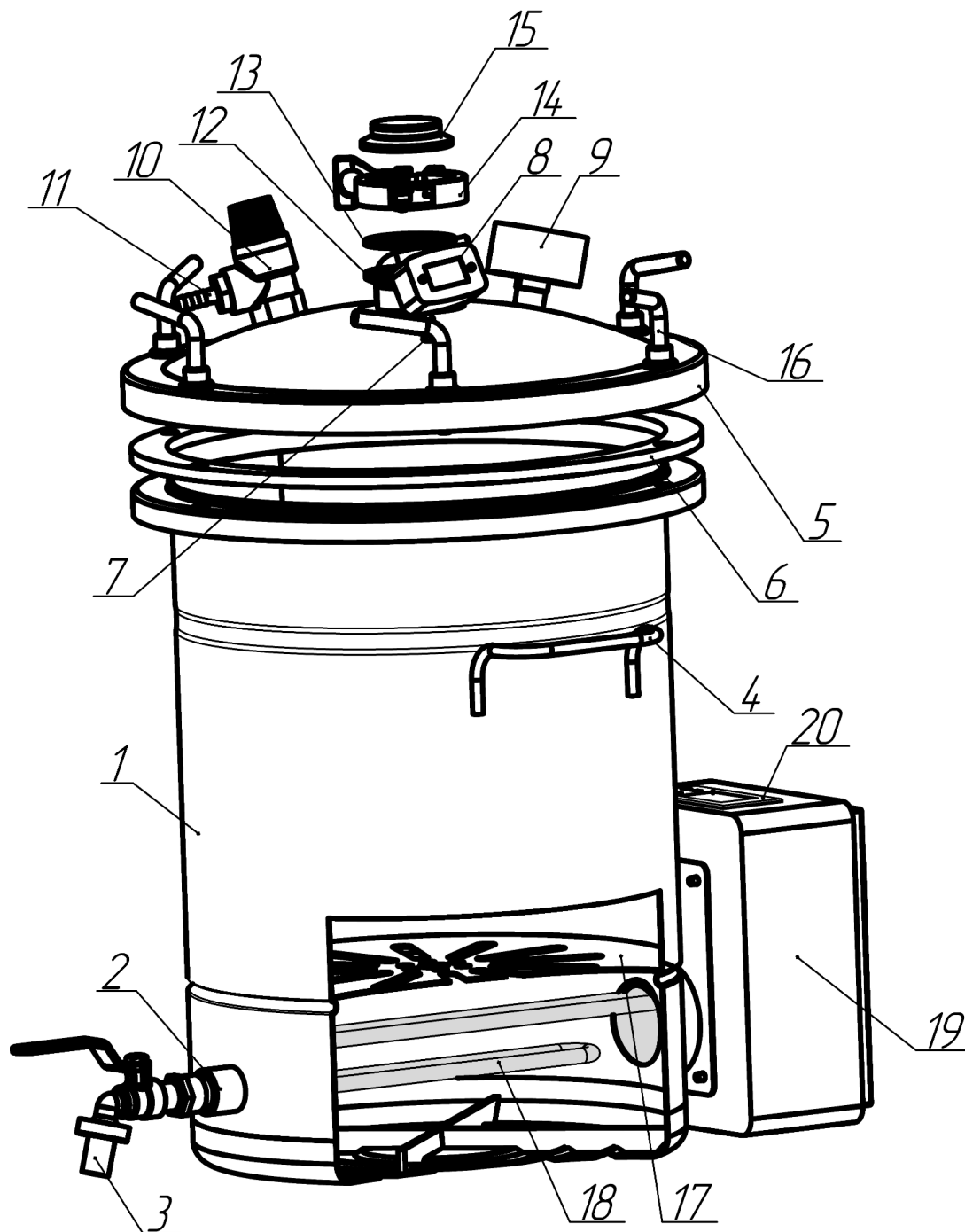
Рисунок 1 - Комплектация автоклава «Булат»
